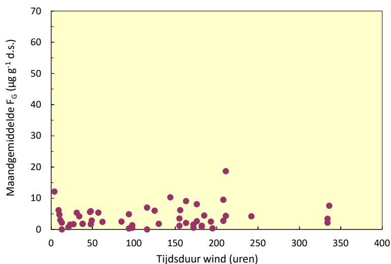
Figuur 8 Voor seizoeninvloeden gecorrigeerde maandgemiddelde fluoridengehalten in gras ( \mu\text{g g}^{-1} d.s.) in relatie tot het aantal uren dat er gedurende de expositieperioden van vier weken wind heeft gewaaid uit de richting van de REC naar de meetpunten rond de installatie. Door de correctie voor verschillen in groeisnelheid worden gehalten in de winterperiode iets lager en in de zomerperiode iets hoger dan gemeten.
