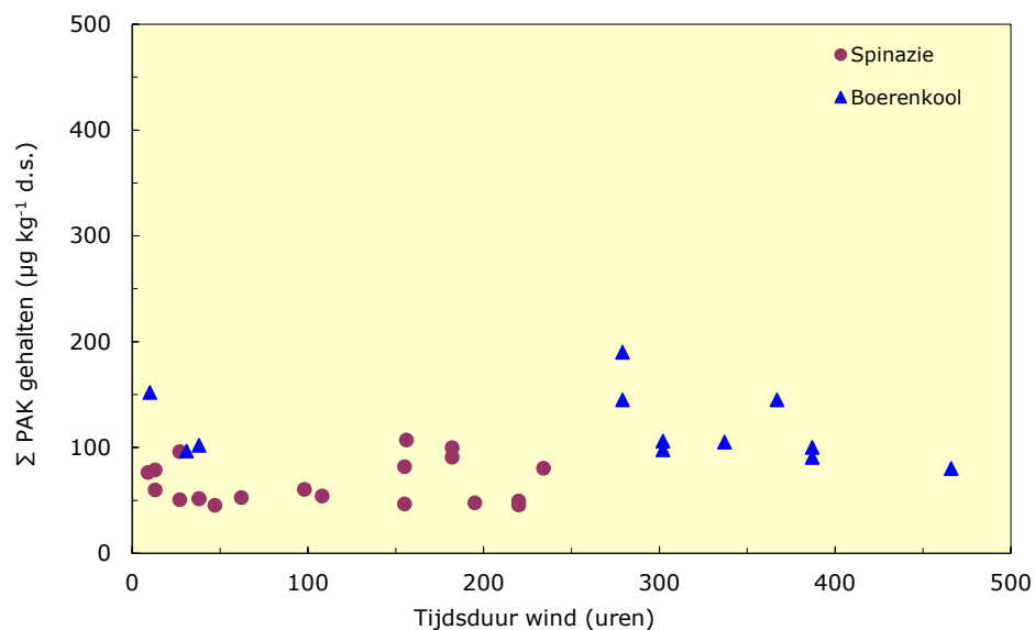
Figuur 4 Totaal PAK-gehalte in spinazie en boerenkool ( \mu\text{g kg}^{-1} \text{ d.s.} ) in relatie tot het aantal uren dat er gedurende de expositieperioden wind heeft gewaaid vanuit de richting van de REC naar de afzonderlijke meetpunten.
