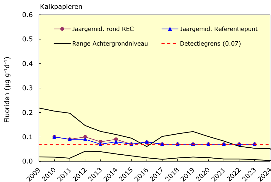
Figuur 7 Trendmatig verloop van het gemiddelde fluoridgehalte in kalkpapieren ( \mu\text{g g}^{-1}\text{d}^{-1} ) in de directe omgeving van de REC en het referentiepunt buiten de directe invloedssfeer van de installatie. De zwarte lijnen geven een indicatie van de bandbreedte van het achtergrondniveau weer, deze berekende waarden liggen inmiddels beneden de detectiegrens (zie Bijlage 1). NB. In 2010 was de REC nog niet operationeel.
